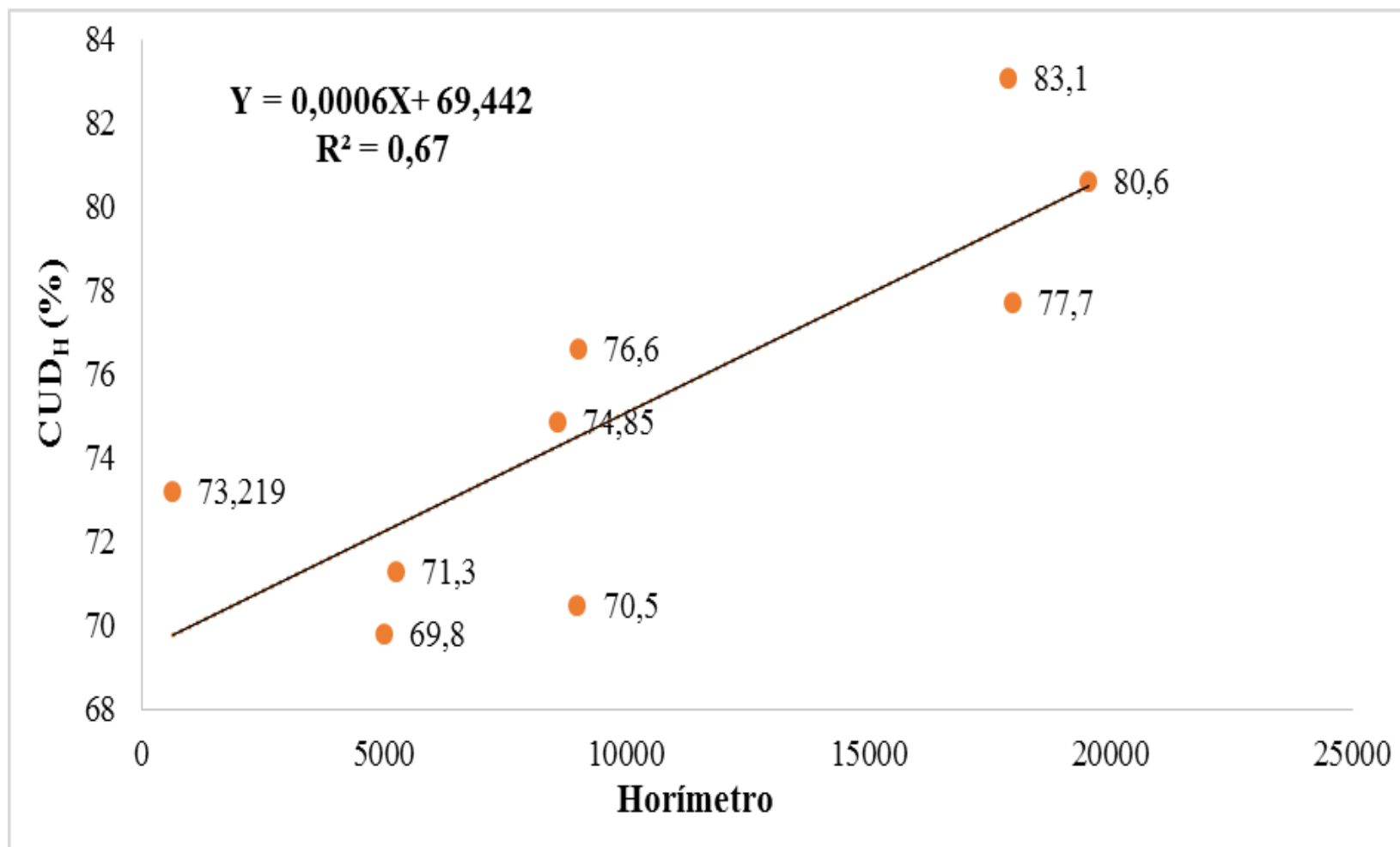
Figura 19- - Coeficiente de Uniformidade e Distribuição em função do tempo de uso.
