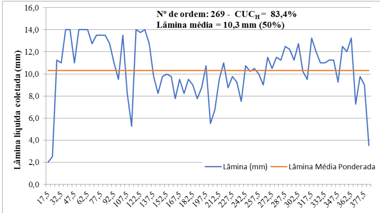
Figura 14- Perfil da lâmina coletada no equipamento 269.
